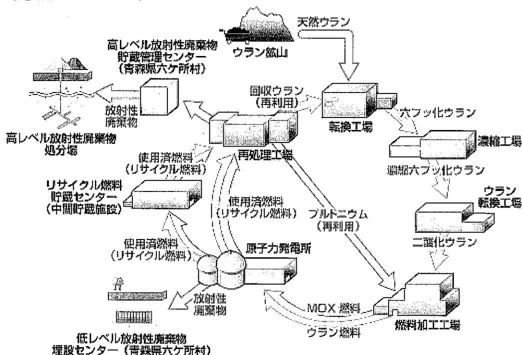
原子燃料サイクル図
