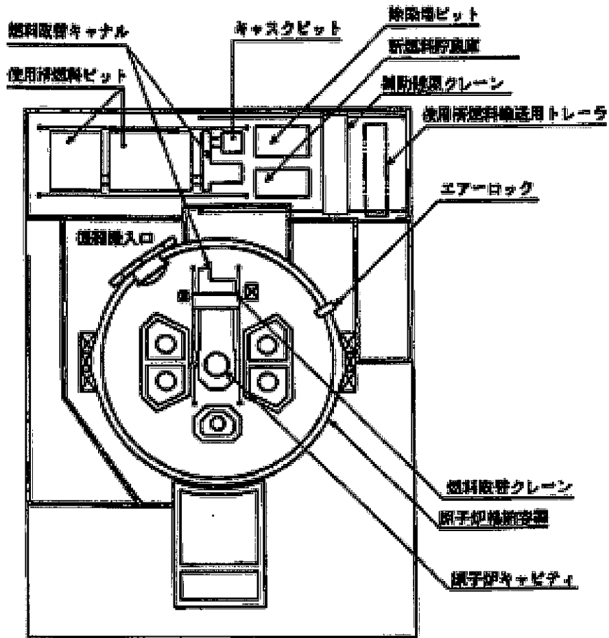
出典：大飯発電所原子炉許可申請書（3，4号炉完本）添付書類八 第6.7.1図 燃料取扱設備配置図
