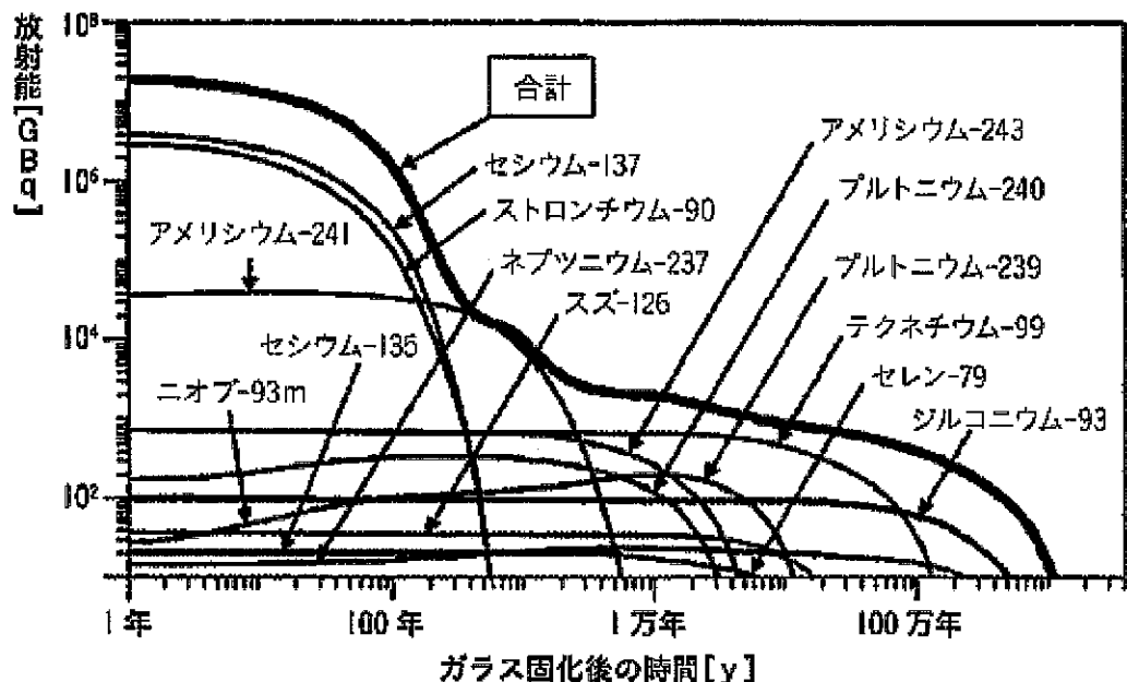
出典：館野淳「シビアアクシデントの脅威」 図5-2 ガラス固化体にした後の放射能強度の時間変化
